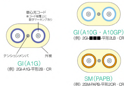
■構造図
