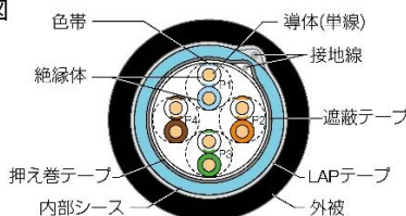
■構造図
