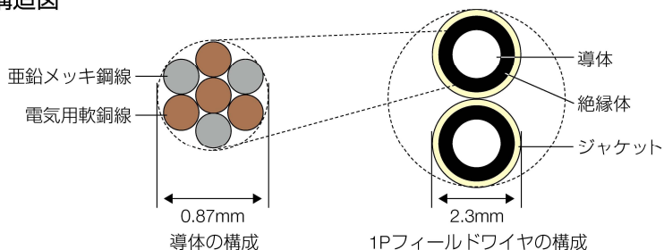
■構造図
