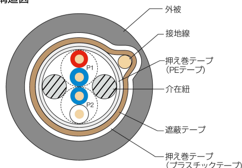
■構造図
