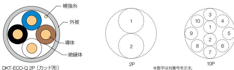
DKT-ECO-Q 2P (カッド形)
