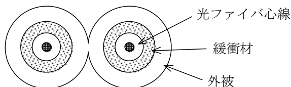
図-1 2心光コードの構造
