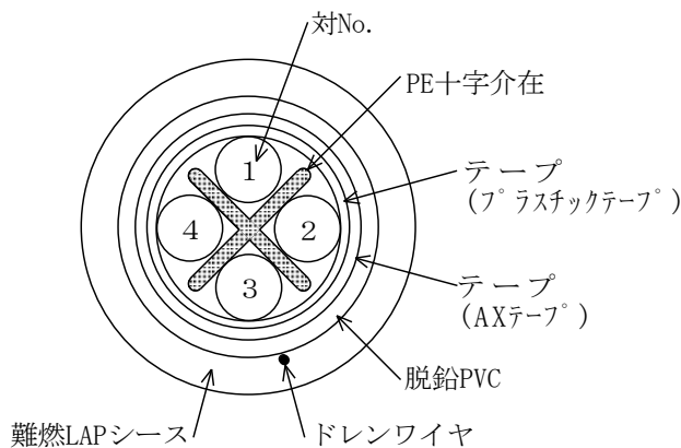
図-1 ケーブルの構成
