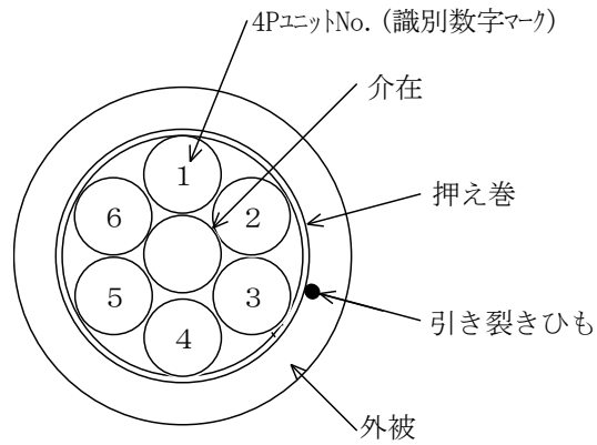
図-2 ケーブルの構成
