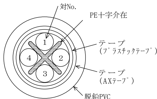
図-1 4Pユニットの構成
