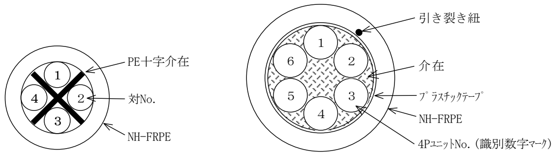
図-1 4Pユニットの構成
