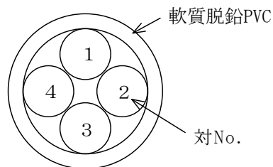
図-1 ケーブルの構成
