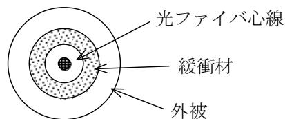
図-1 ECO単心光コードの構造
