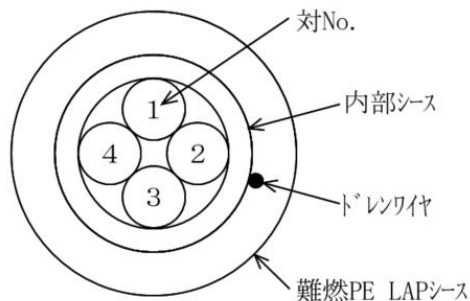
図-1 ケーブルの構成
